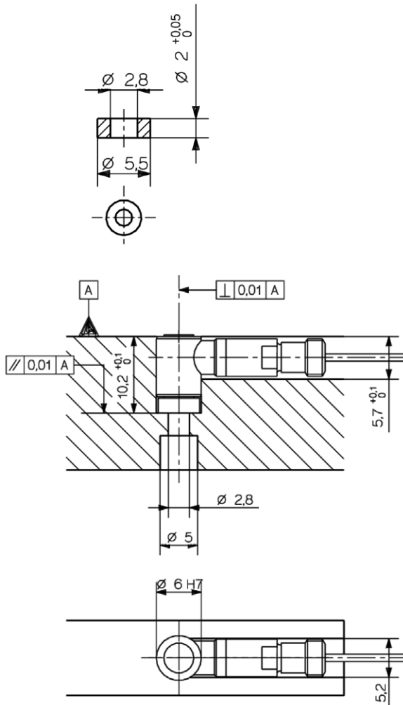
Abb. 1: Einbau in Sackloch mit gehärteter Druckscheibe \varnothing 5,5 Typ 9413
