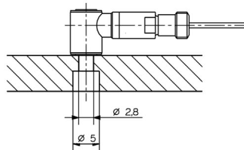
Abb. 2: Einbau in Halteplatte
