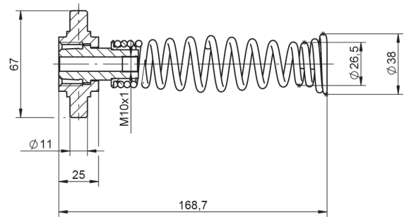
図 3a: トムソンアダプタ 型式 6513A
