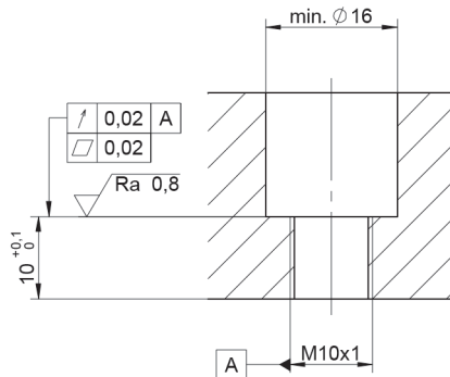
図 1: フラッシュ実装用取付け穴 (4ストローク)
