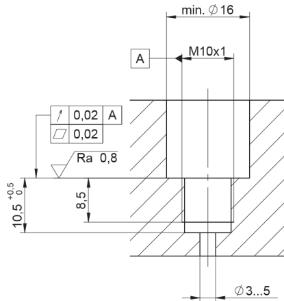
図 2: 追加のガスチャンネルを使用したリセスマウント用の取付け穴 (4ストローク) 取付け穴の長さはアプリケーションにより異なります。取付け穴が長すぎる場合、測定結果に影響を及ぼす可能性があります。
