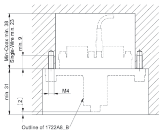
Bild 3: Einbaumasse 8-Kanalstecker Typ 1722A8_B
