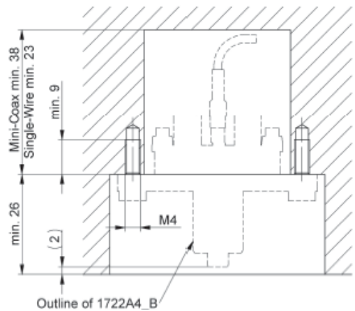
Bild 2: Einbaumasse 4-Kanalstecker Typ 1722A4_B
