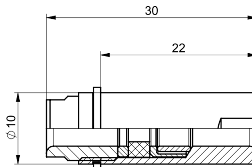
図 13: アダプタ型式1700A37C (鋼製メッシュ付きケーブル用)
