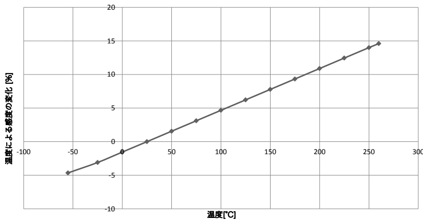
図4: 代表的な温度による感度変化
