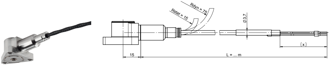
図 5: 8205BxxBDJxx: ケーブル保護なし
