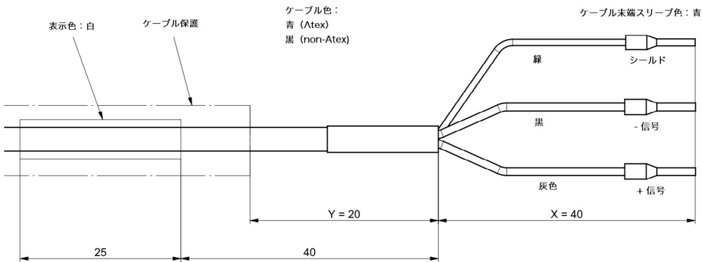
図 9: ケーブル終端処理
