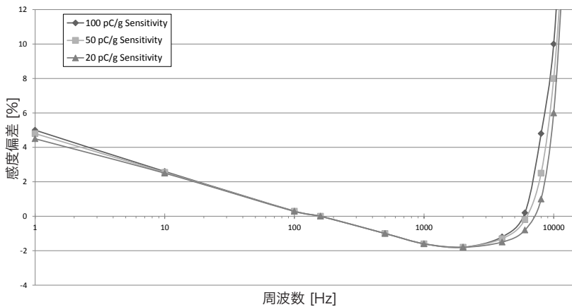
図 3: 代表的な周波数応答: 基準値159Hzに対する
