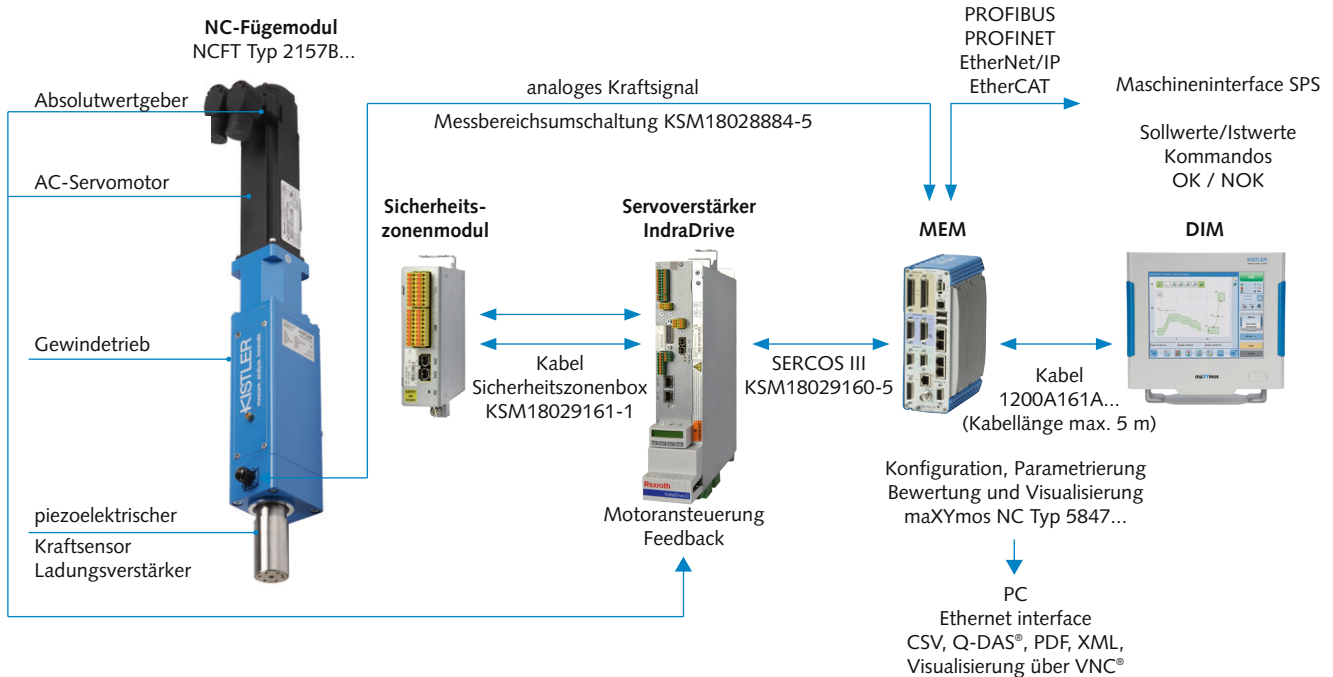
Bild 5: Funktionsprinzip eines NC-Fügesystems mit NC-Fügemodul NCFT Typ 2157B... und maXYmos NC Typ 5847...
