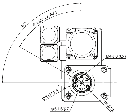
Bild 4: Abmessung Ansicht A, NC-Fügemodul NCFT Typ 2157B1T250 ... 2157B8T250 für Messbereiche von 0,05 ... 1,5 kN
