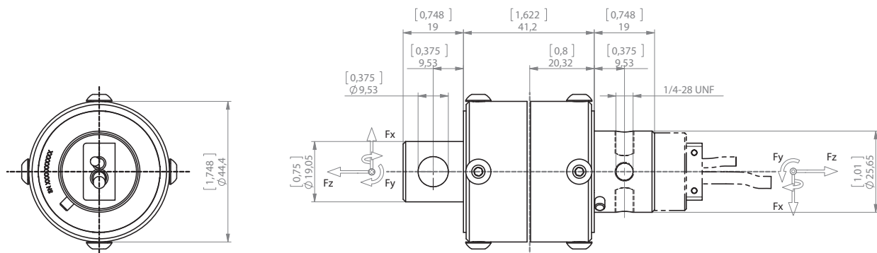
Bild 3: Abmessungen in mm
