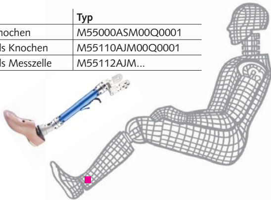
Bild 1: Instrumentiertes Bein und Dummyanwendung
