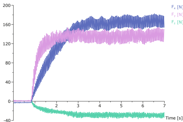
Abb. 2: Messdaten beim Fräsen, erfasst mit DynoWare
