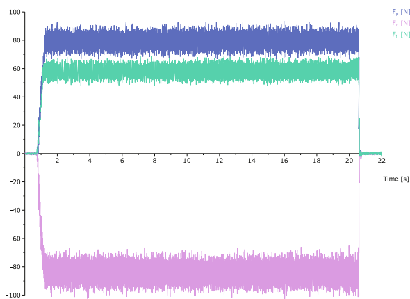
Abb. 1: Messdaten beim Drehen, erfasst mit DynoWare
