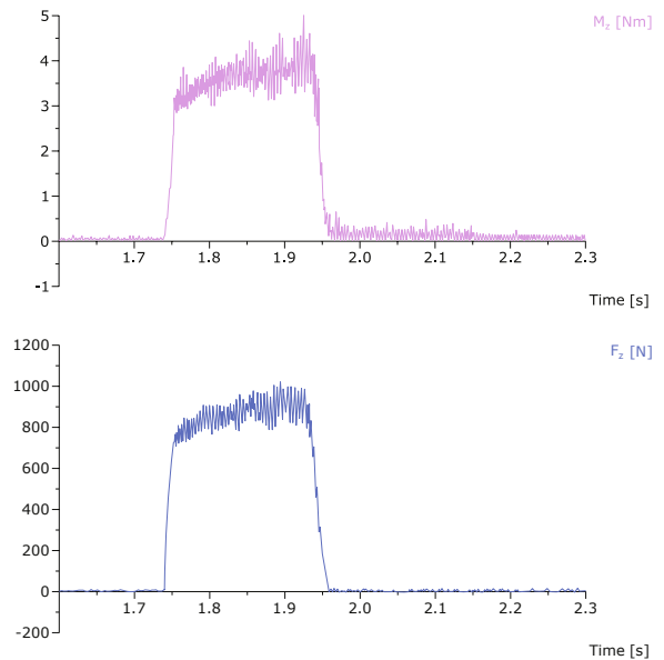
Abb. 3: Messdaten beim Bohren, erfasst mit DynoWare
