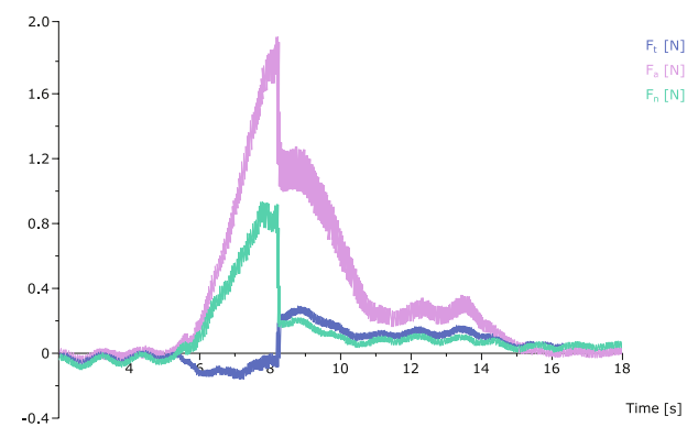
Abb. 4: Bruch der Schleifscheibe beim Schleifvorgang, Messdaten erfasst mit DynoWare
