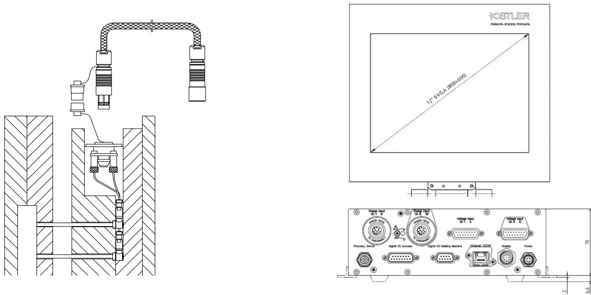
Fig. 3: Capteur Type 9210AA... avec amplificateur de charge Type 5159A...
