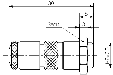
Fig. 10: Connecteur mono-fil Type 1839
