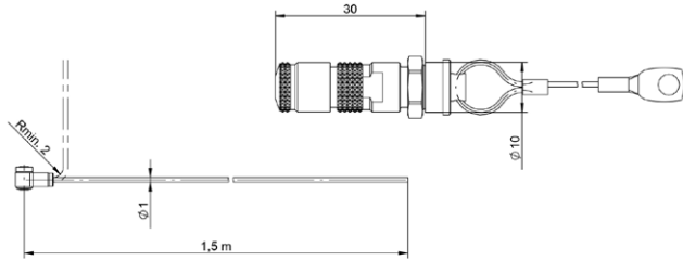
Fig. 1 : Capteur de force type 9210AA avec câble et connecteur
